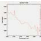
矿产光谱曲线图
