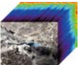
矿产高光谱图
