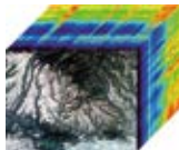
林业高光谱图
