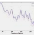
甲烷光谱曲线图
